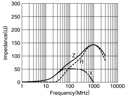
ACZ1005Y-301(MMZ1005Y301C)
