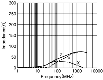
ACZ1005Y-241(MMZ1005Y241C)
