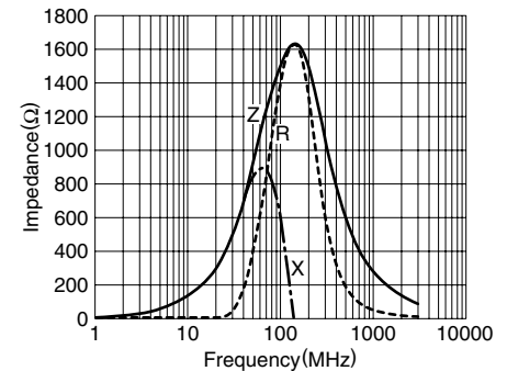
ACZ1005Y-152(MMZ1005Y152C)
