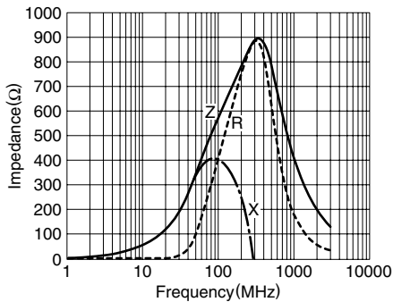
ACZ1005Y-601(MMZ1005Y601C)
