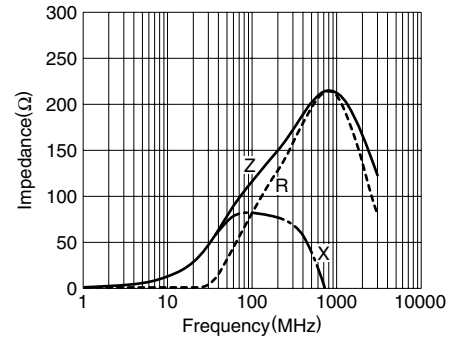
ACZ1005Y-471(MMZ1005Y471C)
